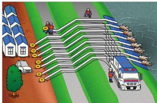
排水ポンプ車 (30m 3 /min)
