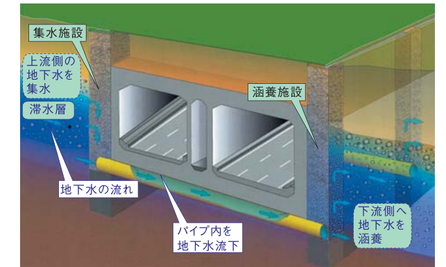
地下水流動保全工法のイメージ図
