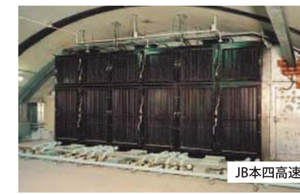
除じん装置の例
