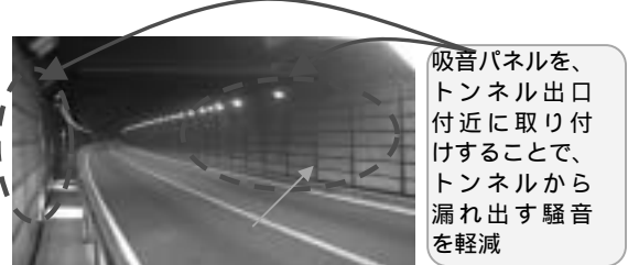
トンネル内の吸音処理
