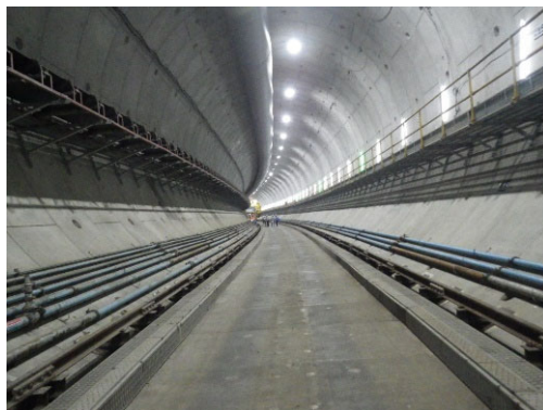
Hランプ坑内(シールド構築状況)
