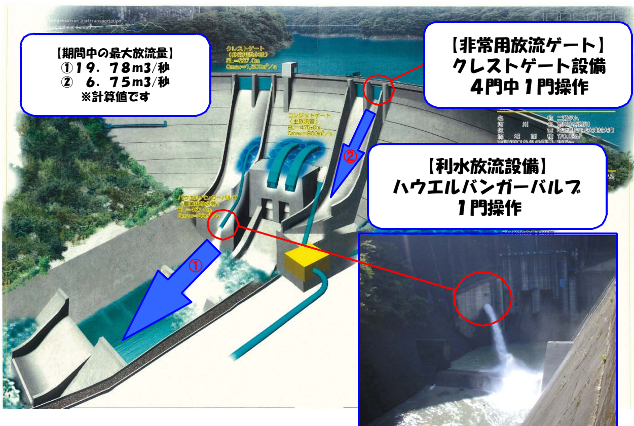
二瀬ダム放流設備
