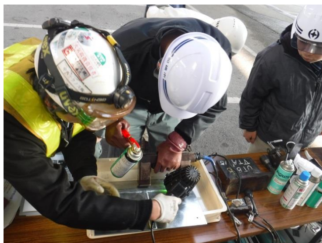
現地実習の状況 (超音波探傷試験)
