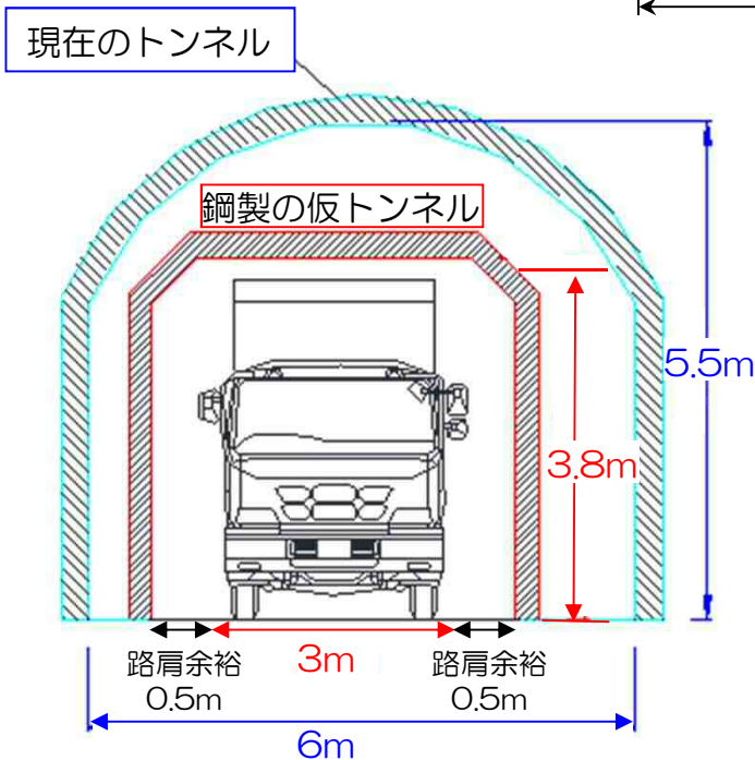
図-2 工事中の断面図
