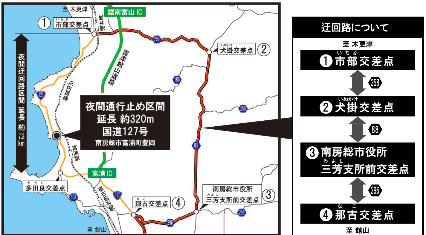
図-4 迂回路位置図
