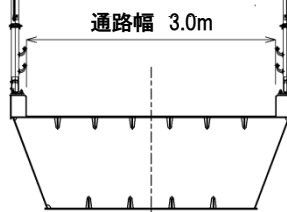
<新設歩道橋>
